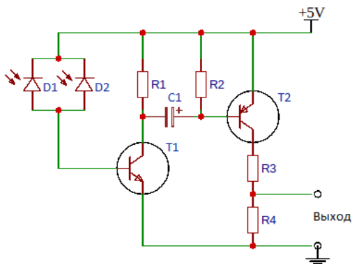
Рисунок 3 — Принципиальная электрическая схема приёмника инфракрасного излучения. Обозначения: D1, D2 – фотодиоды BVP10NF; T1 – транзистор KT3102; T2 – транзистор KT3107; C1 – электролитический конденсатор 10 мкФ; R1, R2 – резисторы 10 кОм; R3 – резистор 20 кОм; R4 – резистор 51 кОм
