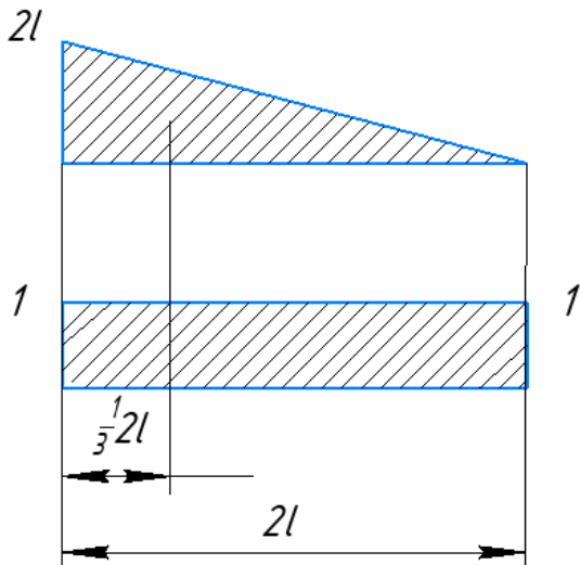
Рисунок 6 — Эпюра моментов при нагрузке системы опорной реакцией x_1 = 1 и опорным моментом x_3 = 1 для определения коэффициента \delta_{31}
