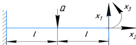
Рисунок 2 — Эквивалентная система
