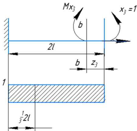
Рисунок 5 — Эпюры моментов при нагрузке системы опорным моментом x_3 = 1
