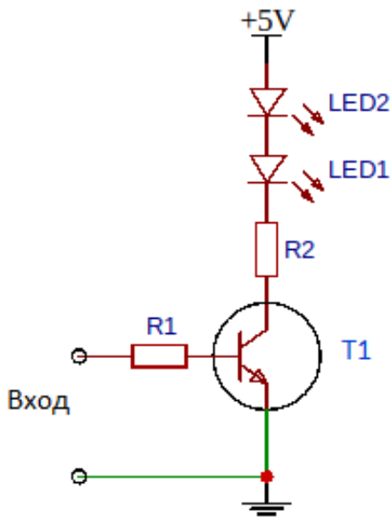
Рисунок 2 — Принципиальная электрическая схема излучателя инфракрасных импульсов. Обозначения: T1 – транзистор KT3102; LED1,LED2 – светодиоды TSAL6100; R1 – резистор 300 Ом; R2 – резистор 10 Ом
