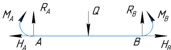
Рисунок 1 — Схема статически неопределимой системы
