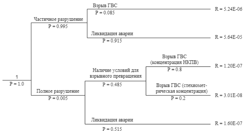
Рисунок 2 — Фрагмент дерева событий для аварии на установке АГРС
