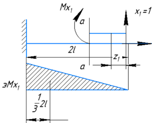
Рисунок 4 — Эпюры моментов при нагрузке системы опорной реакцией x_1 = 1 для определения коэффициента \delta_{11} .
