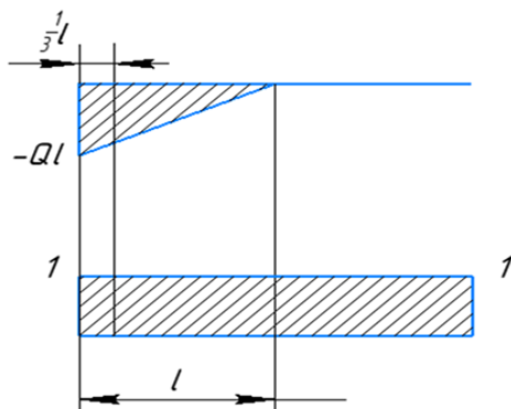
Рисунок 9 — Эпюры моментов M_{xp} и M_{x3} для определения коэффициента \Delta_{3p}
