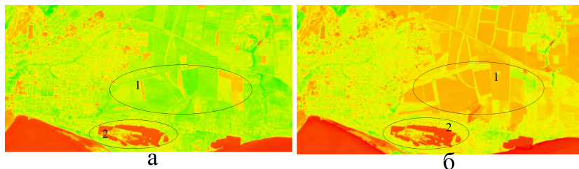
Рисунок 2 — Результат обработки изображений с использованием индекса NDVI на почвах подтвержденных засолению
